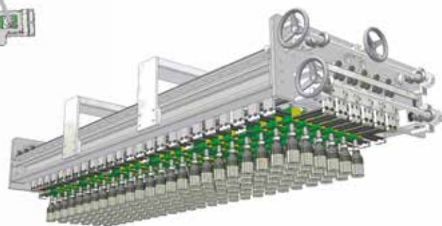
Универсальная головка с долговечными захватными патронами
