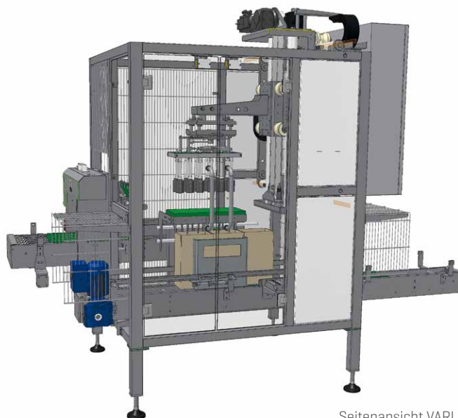
Seitenansicht VARI
