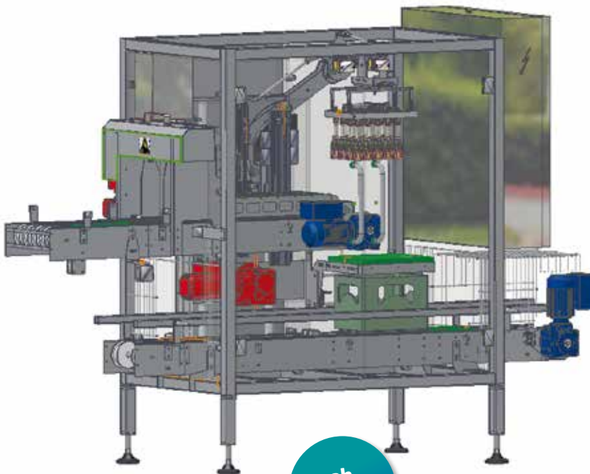
Aus-/Einpackmaschine UNO
